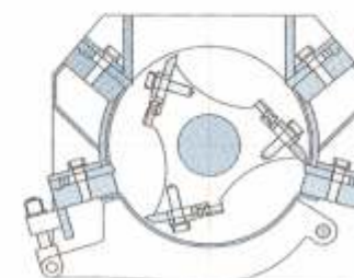
四支固定刀結構示意圖 Structure Diagram of 4 Knives
