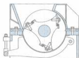
兩支固定刀結構示意圖 Structure Diagram of 2 Knives
